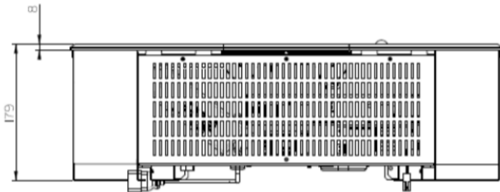
SCALE 0.250
